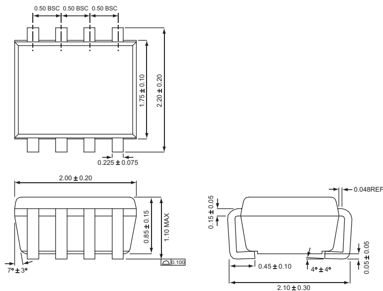
SC70JW-8
